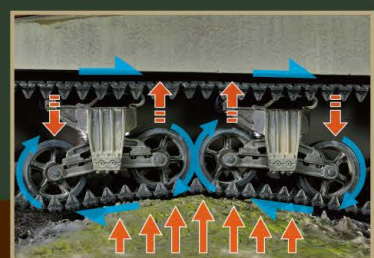
滚动路轮及真实的垂直螺旋弹簧悬吊系统。
