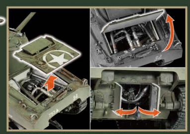
可拆装及开关的发动机舱门。
