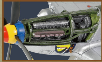
• 发动机结构细节
