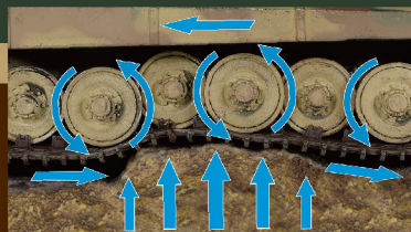
活動式悬架及车轮可自由转动
