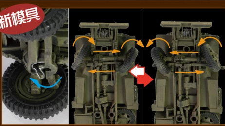
前轮卡扣锁-解锁后能随意调整车轮转向
